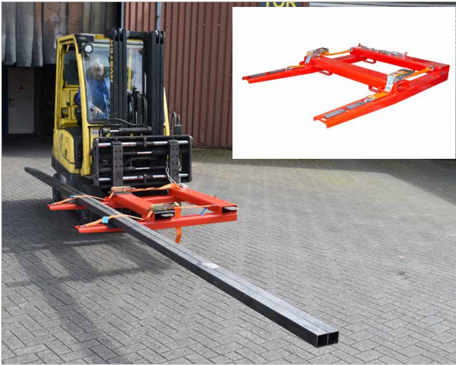
Aufnahmeposition zum Transport z.B. durch Tore oder Gänge
