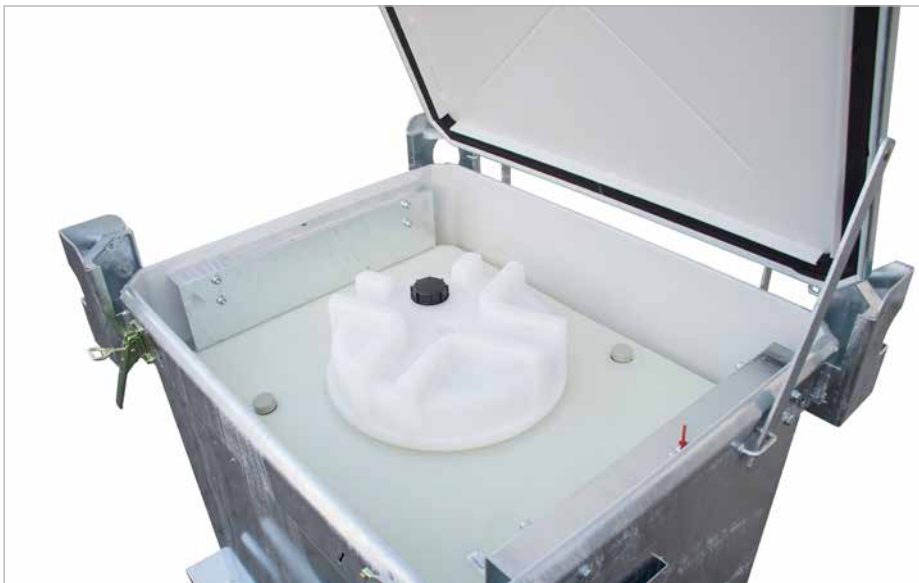
Stahl-Außenbehälter und PE-Innenbehälter mit Schraubdeckel
