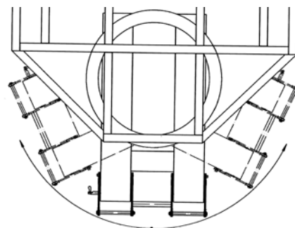
Drehkranz mit Einfahrtaschen
