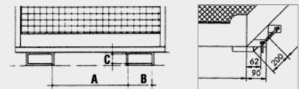
Einfahrtaschen-Innenmaße (mm)
